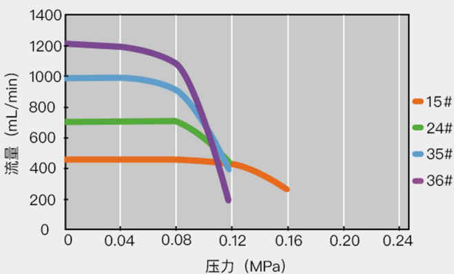
DY25泵头压力/流量曲线图（100rpm）
