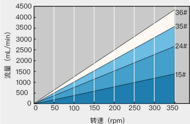
DY25泵头流量范围（0.1–350rpm）
