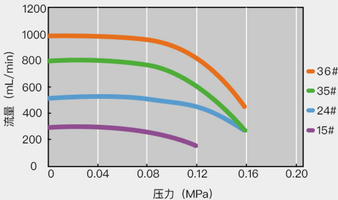
DZ25-6L泵头压力/流量曲线图 (100rpm)
