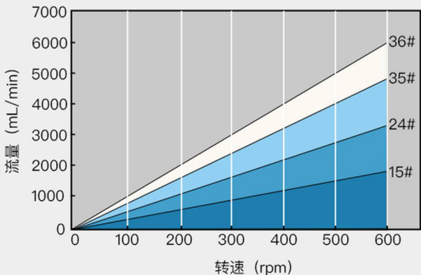
DZ25-6L泵头流量范围 (0.1-600rpm)
